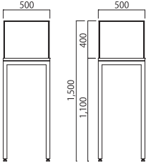
展示ケース・STC-5050
