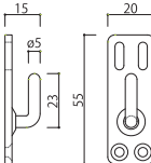
FHO-55 φ3.8—11.8長穴×2ヶ所 φ4穴—φ7.2皿×2ヶ所
