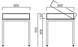
展示ケース・STF-8080
