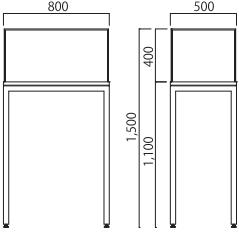
展示ケース・STC-5080
