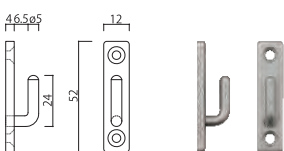
FHO-52SG φ4穴—φ8皿×2ヶ所
