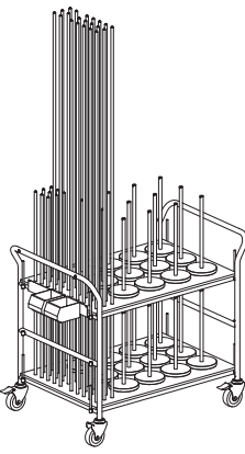
NT-WGK-2 (フレキシブル40・フラットバー40タイプ) 専用ワゴン (詳細は、P69参照)
