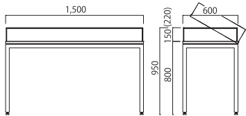
展示ケース・STF-15060 (15060-2)
