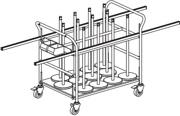
NT-WGK-3 (フレキシブル75・フラットバー72タイプ) 専用ワゴン (詳細は、P69参照)
